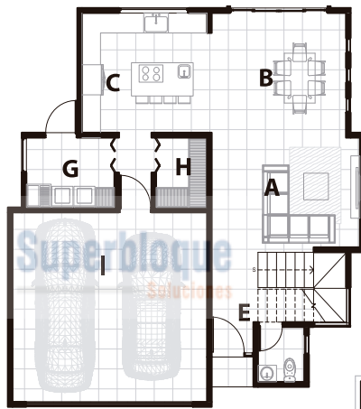
NIVEL 1
