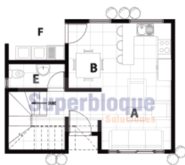
NIVEL 1
